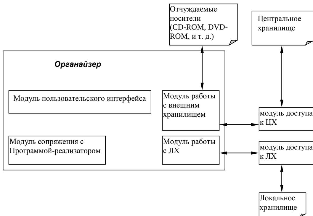
Рис.5. Структура приложения «Организер»
