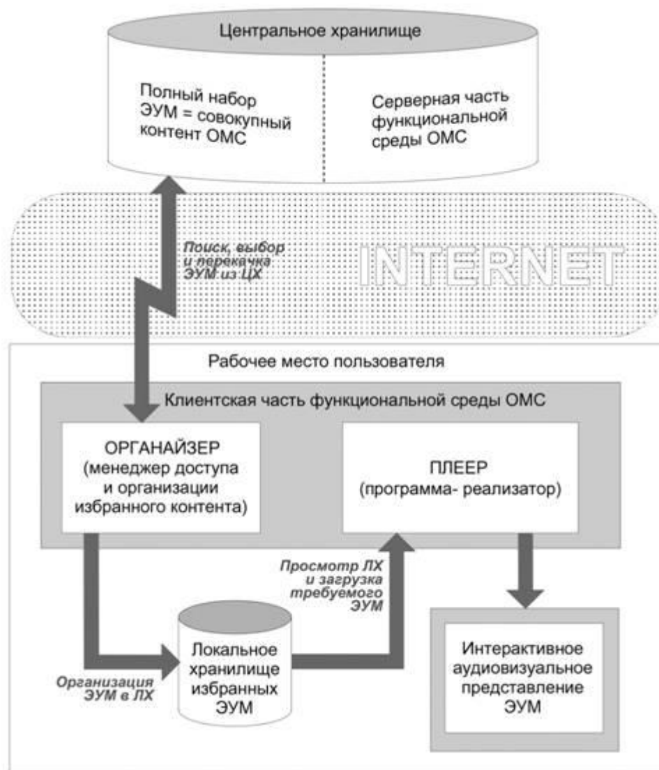
Рис. 3. Общая архитектура ОМС
